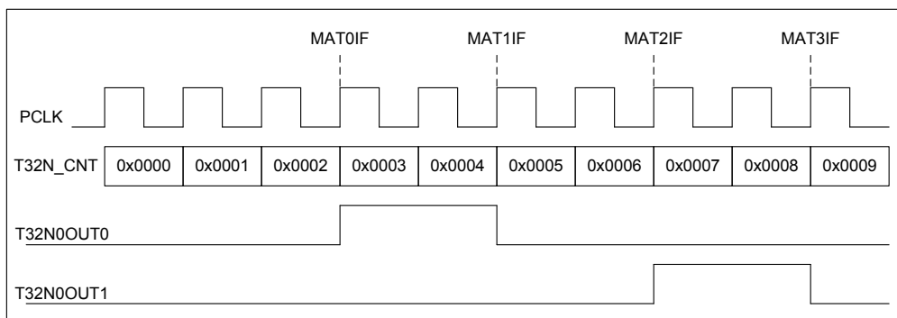
图 5-10 T32N0 输出调制功能示意图
