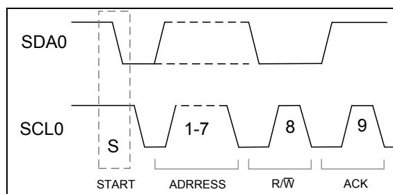
图 5-38 I2C 起始位波形图
