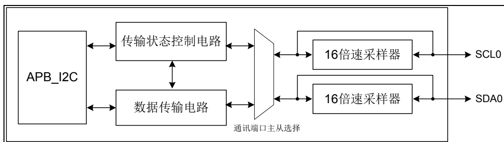
图 5-30 I2C 电路结构框图
