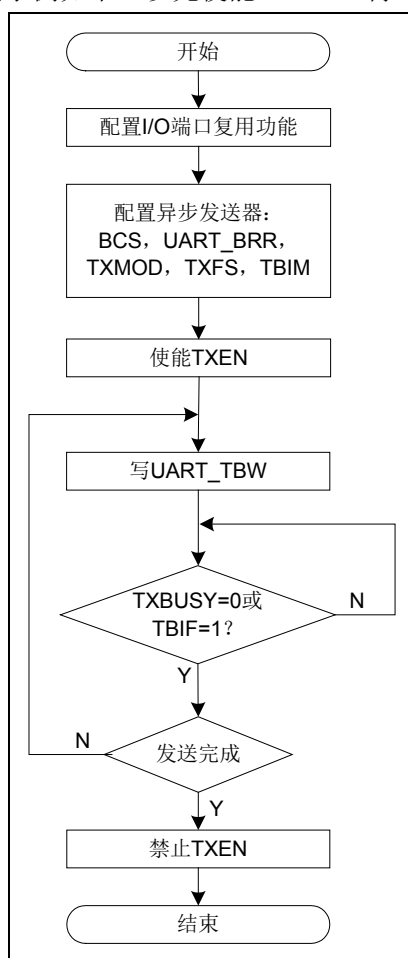
图 5-16 UART 发送数据操作流程图示例
