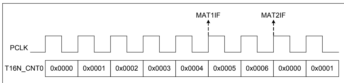
图 5-2 T16N0 计数匹配功能示意图
