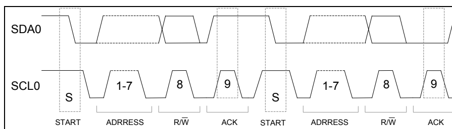
图 5-39 I2C 自动寻呼波形图
