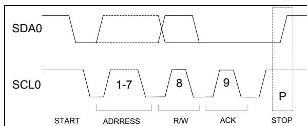
图 5-40 I2C 停止位波形图
