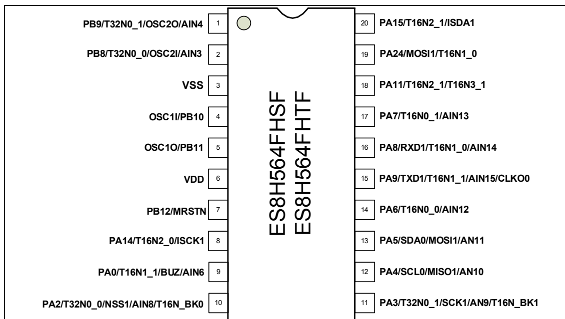
图 1-2 SOP20/TSSOP20 封装顶视图
