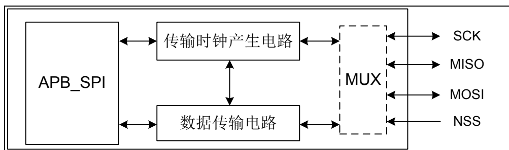
图 5-22 SPI 电路结构框图
