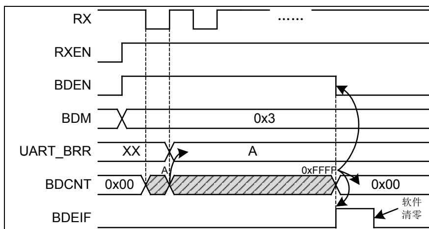
图 5-20 自动波特率检测错误时序示意图
