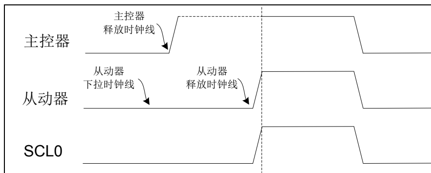
图 5-43 I2C 时钟线下拉等待波形示意图
