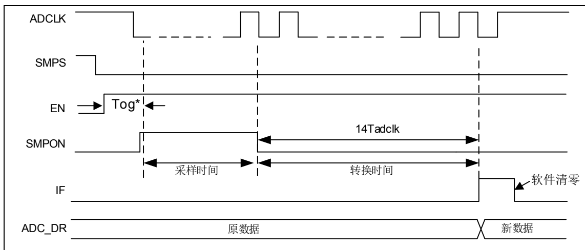
图 5-45 ADC 数据转换时序示意图 (ADC_CON1 寄存器的 SMPS=0, 软件控制采样)
