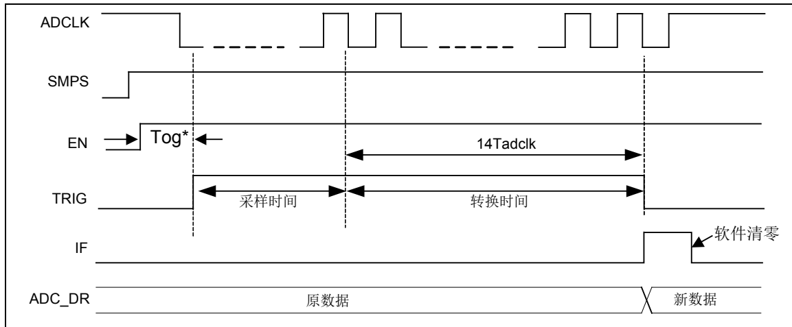
图 5-46 ADC 数据转换时序示意图 (ADC_CON1 寄存器的 SMPS=1, 硬件控制采样)
