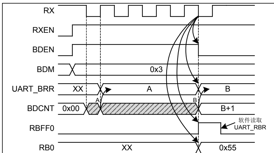
图 5-19 自动波特率检测时序示意图
