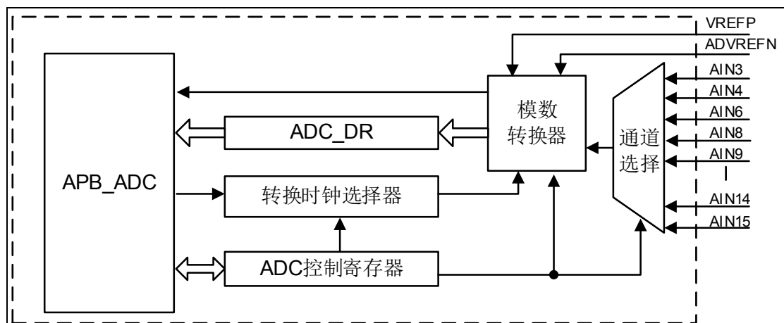
图 5-44 ADC 内部结构图
