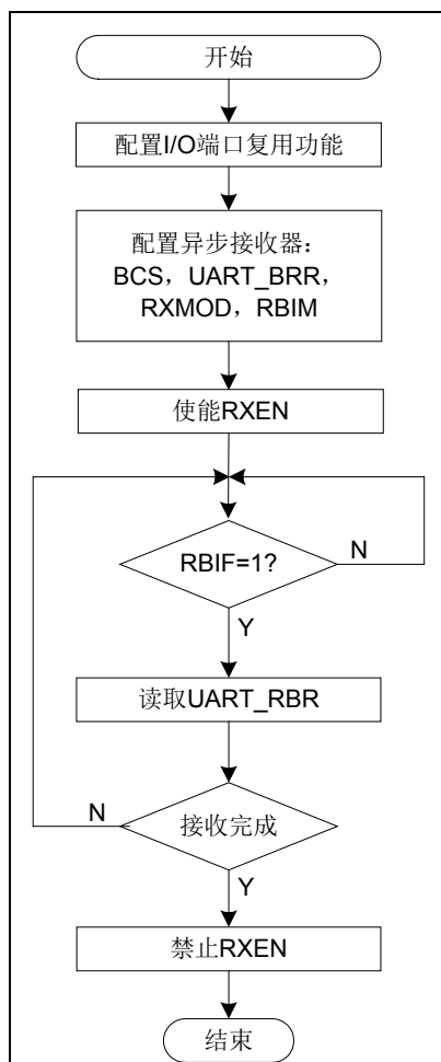
图 5-18 UART 接收数据操作流程图示例
