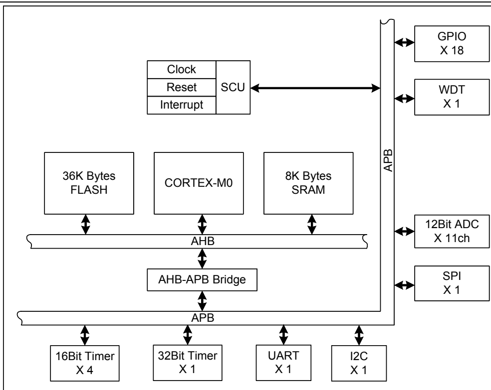
图 1-1 ES8H564 结构框图
