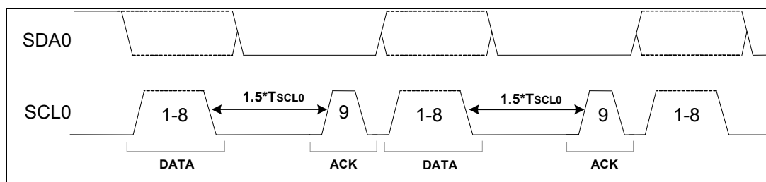
图 5-41 I2C 应答延迟功能波形示意图
