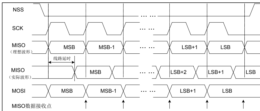
图 5-29 SPI 延迟接收功能波形示意图
