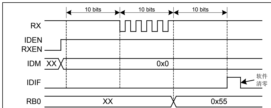
图 5-21 空闲帧检测时序示意图
