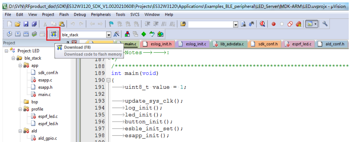
图 2-17 下载
