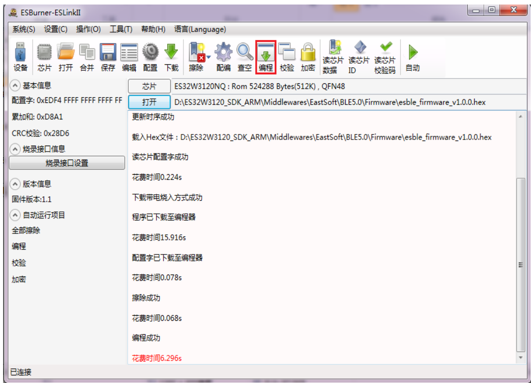
图 2-15 编程
